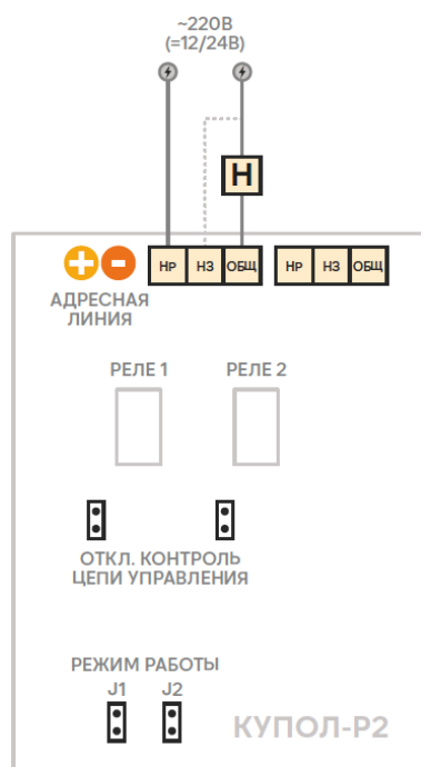
Рис.2. Расположение клемм и органов управления КУПОЛ-Р2. Схема подключения нормально-выключенной нагрузки.
